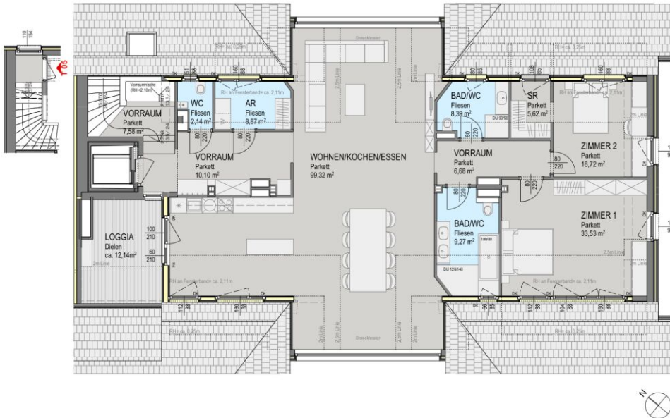
Grundriss Dachgeschoss
