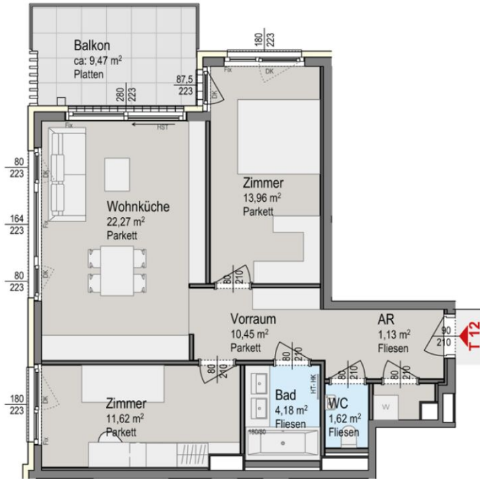
Grundriss 1. Obergeschoß
