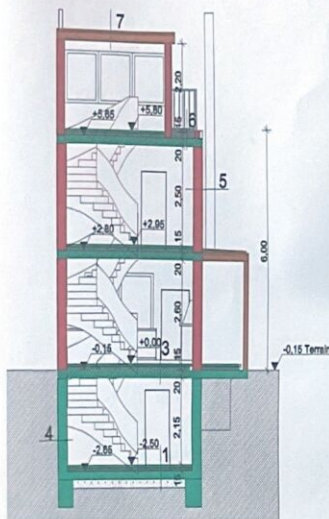
SCHNITT A-A
