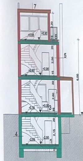
SCHNITT A-A
