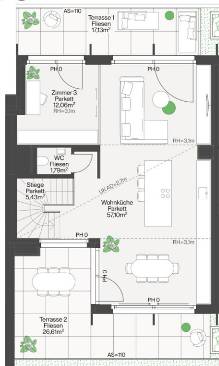
5. Obergeschoß
