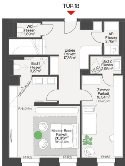
4. Obergeschoß
