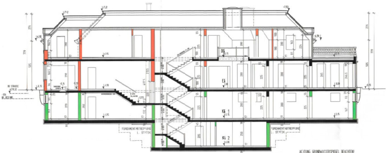
SCHNITT A-A
